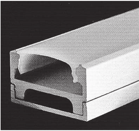
LED-Profil12 mit Profil12f + Profil12m
